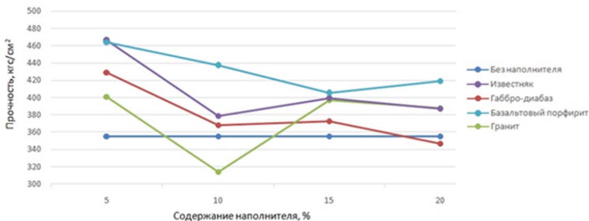
Рис. 2. Зависимость прочности выдерживаемой образцами бетона, от количества наполнителя
