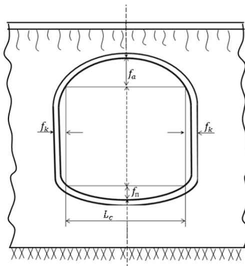
Рис. 1. Конструкция подземного перехода
