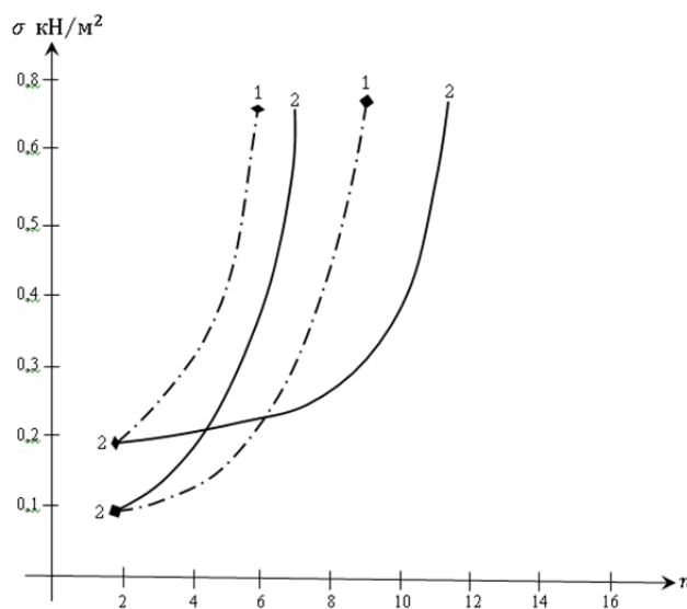
Рис. 3. Изменение напряжения в сооружении от числа -n точек от начала координат 1 – грунт – глина; 2 – грунт – супесь; сплошная линия – теоретические расчеты. прерывистая линия – результаты экспериментов.
